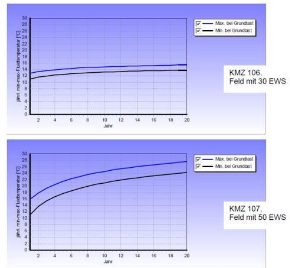
Produktionsstandort der Leica Camera AG Wetzlar mit EED-Berechnungen für die beiden Sondenfelder
